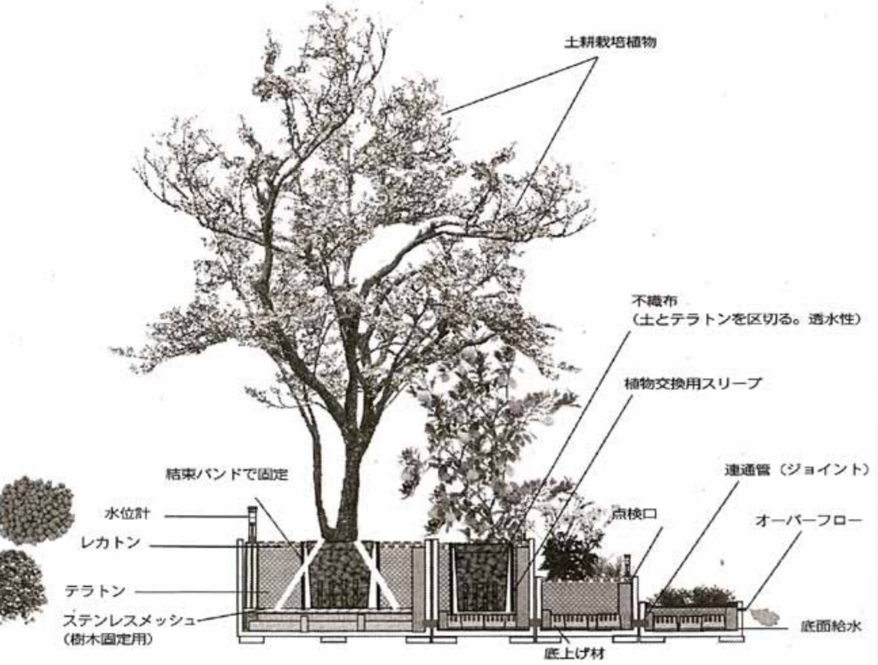
コンポガーデンシステム断面図
